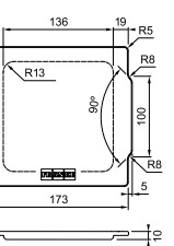
Wooden bowl lid
